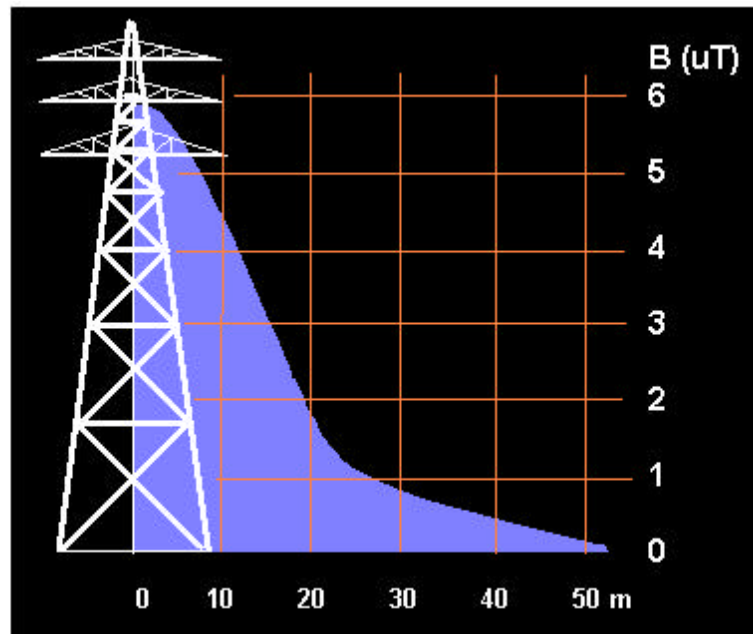
Figura 5. Valores de inducción magnética (en micoteslas, \mu\text{T} ) medidos a 1 metro de altura sobre el suelo, en las cercanías de una línea de transporte eléctrico (la torre no está representada a escala). Se observa que los valores de B se reducen significativamente al aumentar la distancia a la línea. Así, en la vertical de la línea, B podría alcanzar valores de hasta 6 \mu\text{T} ; a 15 metros de la línea, B se reduciría a la mitad, y para distancias superiores a 30 metros B estaría en el orden de las décimas del microtesla. El Consejo de Ministros de Sanidad de la Unión Europea recomienda que el público no esté expuesto a niveles de B superiores a 100 \mu\text{T} .
